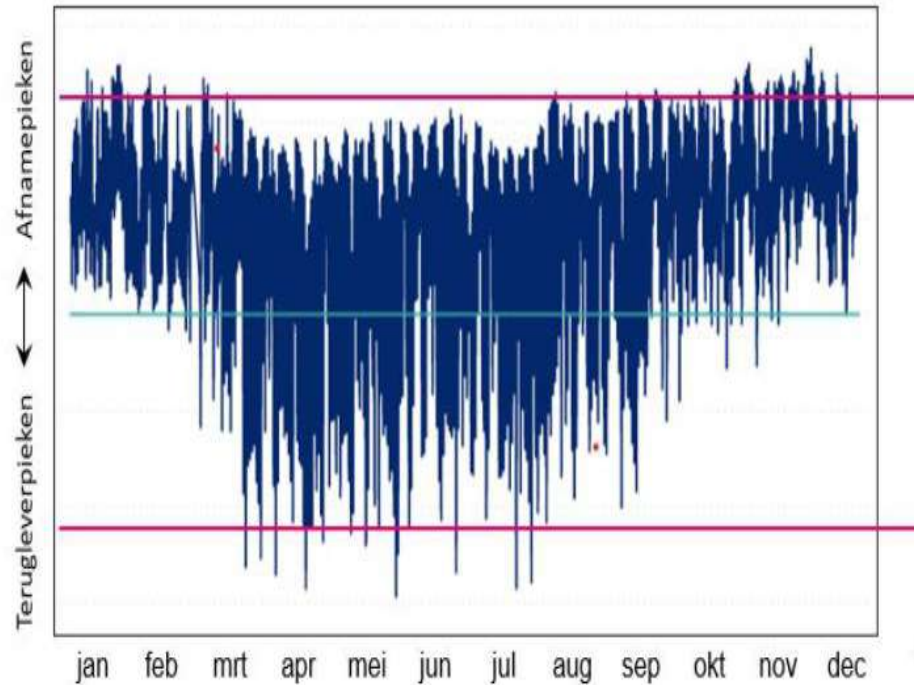
Jaarprofiel HS/MS-station (fictief voorbeeld)
