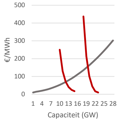
Klassieke merit order
